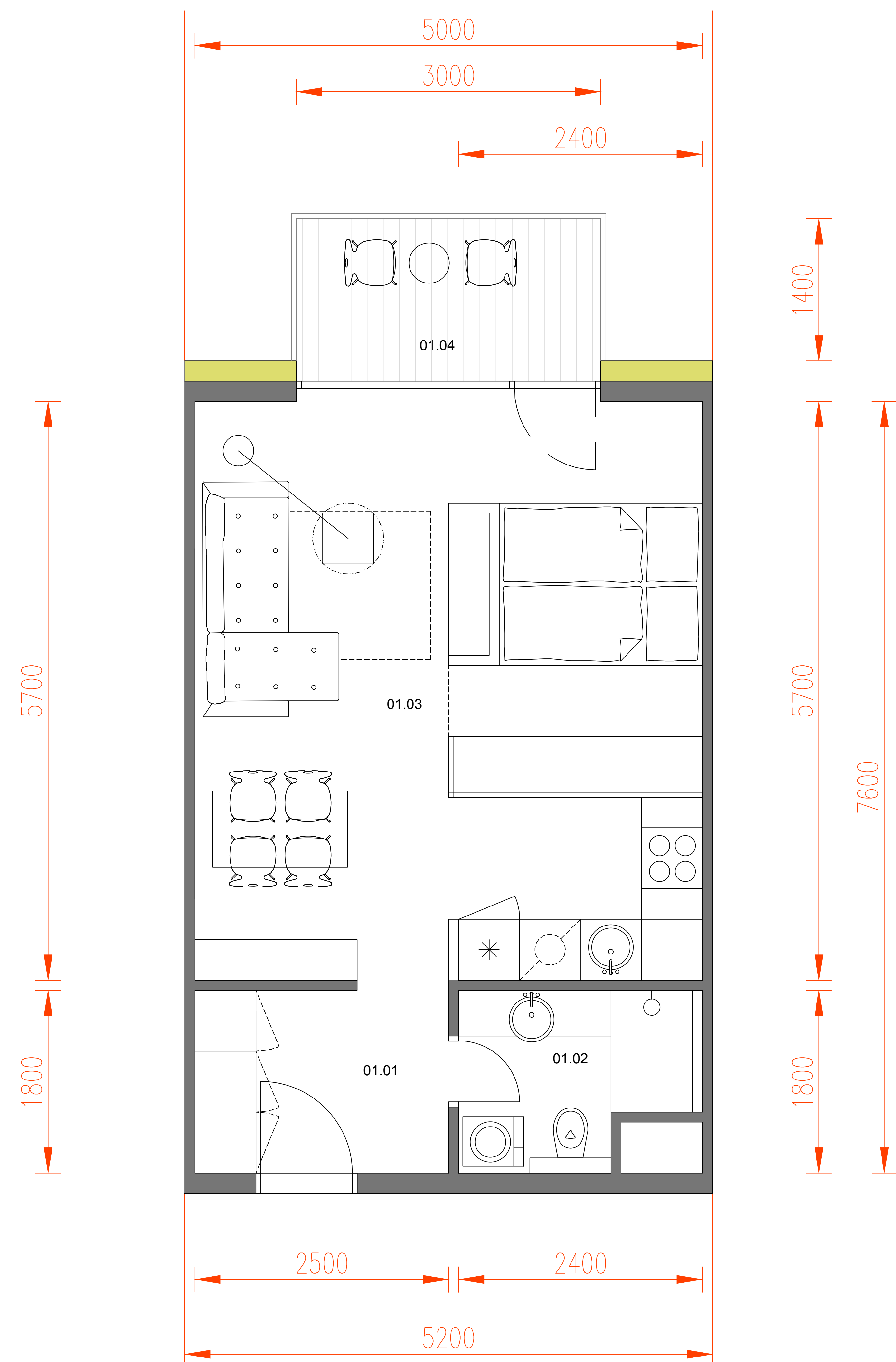
pôdorys 1,5i,modul 5,2m 36,66m2 + 4,80m2
